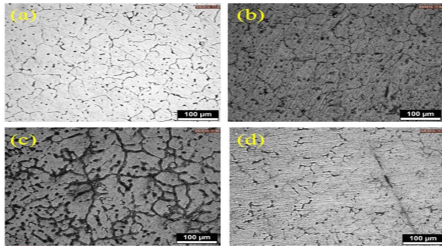
Figure 4.4 Optical microstructure of (a) AST0, (b) AST5, (c) AST10 and (d) AST15
